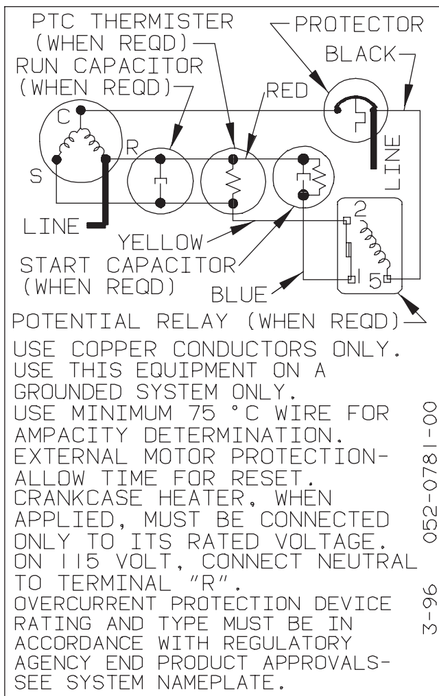
Wiring Diagram 0781
