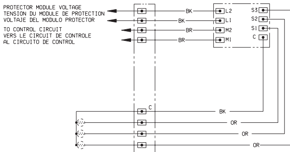
120 OR 240 VOLT MODULE WIRING
