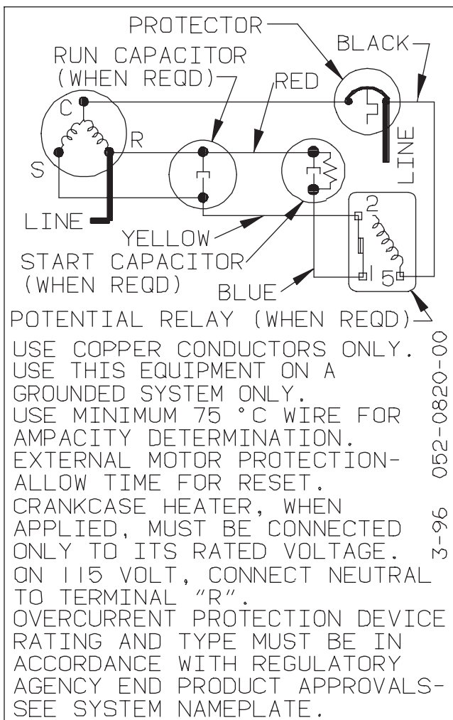
Wiring Diagram 0820
